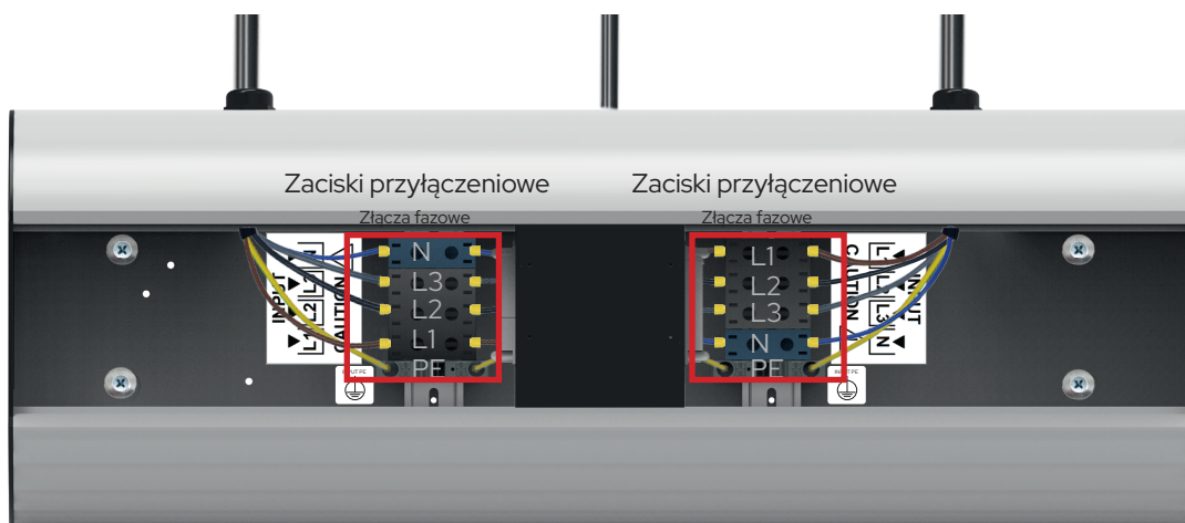
Zaciski przyłączeniowe w ramie Wallbox Frame HT 700
