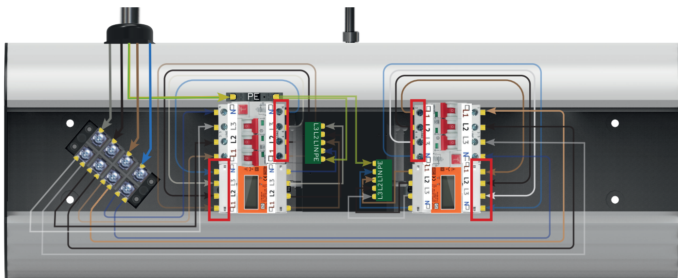
Wallbox Frame HT 700 z kostką przyłączeniową Splitter + RCB O i licznik energii MID.
