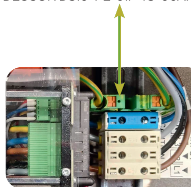
Podstawowa wersja rami Wallbox frame HT 700
