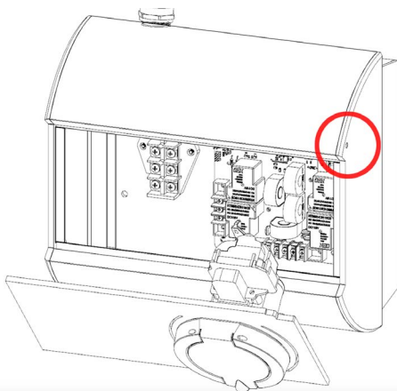
Rys. 53: Punkt pomiaru rezystancji uziemienia obudowy
