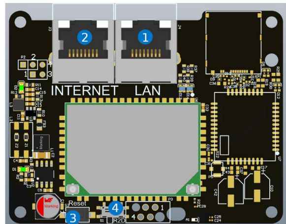
Rys. 24: Budowa Enelion Bridge
