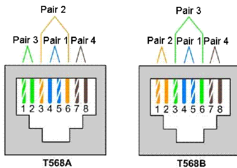
Rys. 52: Zakończenie przewodu Ethernet wg TIA-568A/B do 100BaseT.
