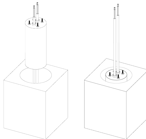
Rys. 23: Posadawianie prefabrykatu w wykopie.
