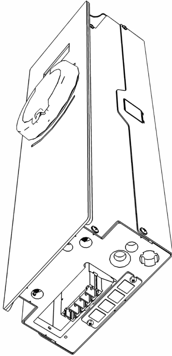
Rys. 11: Moduł ENELION VERTICA kompatybilny ze słupem wyposażonym w moduł ENELION VERTICAN
