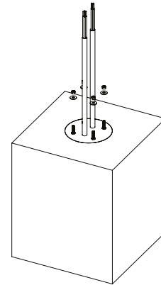
Rys. 35: Wkręcenie nakrętek i podkładek dystansowych na wystające pręty.
