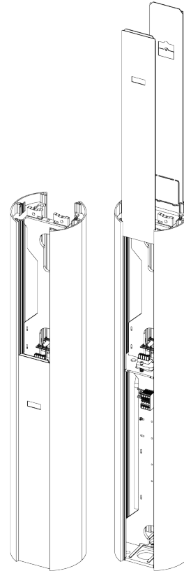
Rys. 36: Wysuwanie dolnych paneli maskujących ze Słupa ENELION VERTICA.
