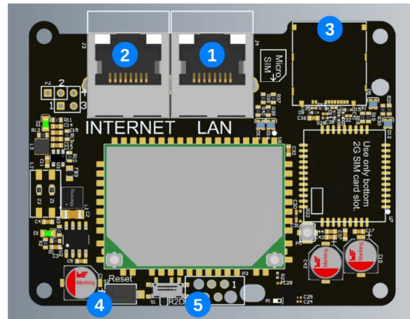
Rys. 54: Schemat modułu ENELION BRIDGE.
