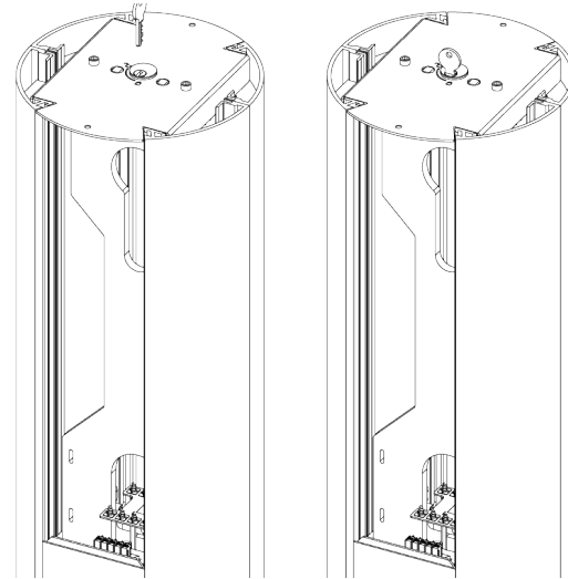
Rys. 5: Odblokowanie płyty zamka.
