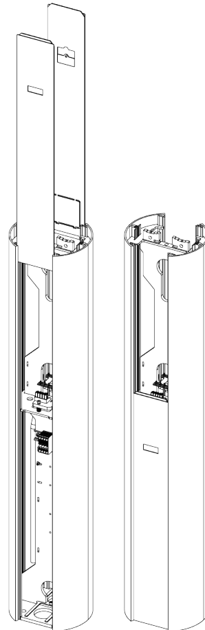
Rys. 67: Rewers Słupa ENELION VERTICA po zamontowaniu ENELION VERTICA Splitter z obecnym licznikiem MID.
