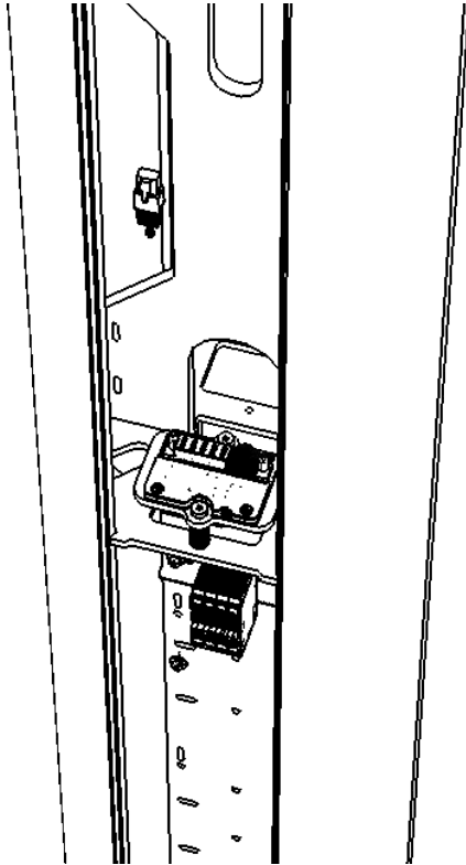
Fig. 64: Lokalizacja ENELION VERTICA link na słupie.
