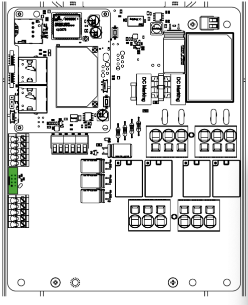
Fig. 29: PilotBox RCM B socket
