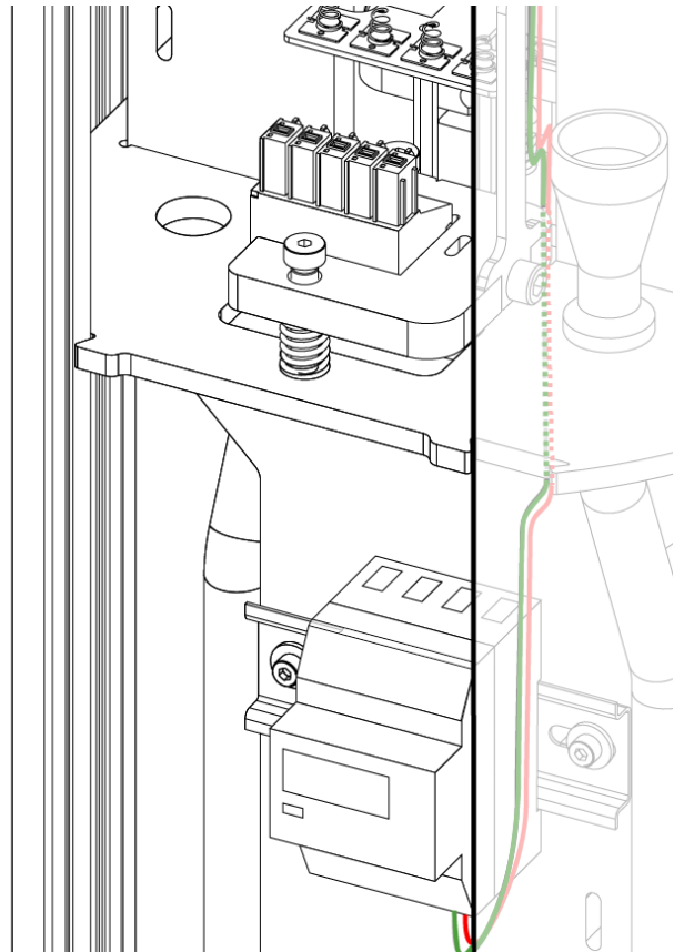
Rys. 58: Lokalizacja ENELION VERTICAN na słupie.
