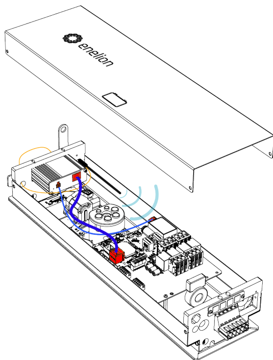
Rys. 76: Prawidłowo zamontowany moduł LTE.
