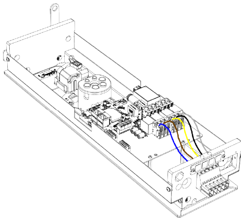
Rys. 69: Odłączyć 4 przewody oznaczone N, L1, L2, L3 ze złącza zasilania. Należy skorzystać ze śrubokręta o zakończeniu PZ2.
