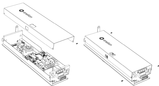
Rys. 67: Zamykanie Modułu ENELION VERTICA.
