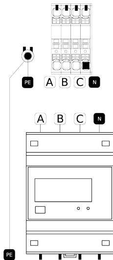
Rys. 42: Schemat relacji pomiędzy podłączeniem standardowym a z zastosowaniem licznika MID.
