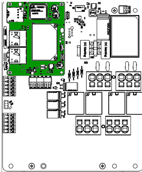
Rys. 66: Dodatek Enelion BRIDGE zamontowany w Module ENELION VERTICA.
