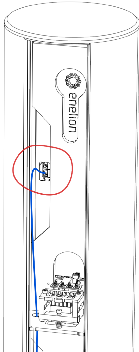
Rys. 51: Przewód poprowadzony do gniazda Ethernet
