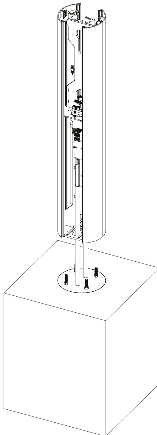
Rys. 36: Osadzony i przykręcony Słup ENELION VERTICA.
