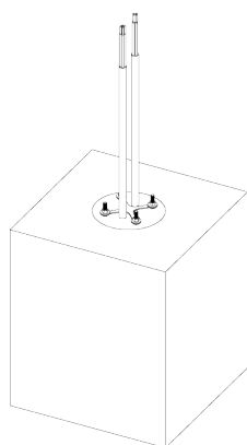
Rys. 30: Poprawnie zabetonowany zestaw fundamentowy.
