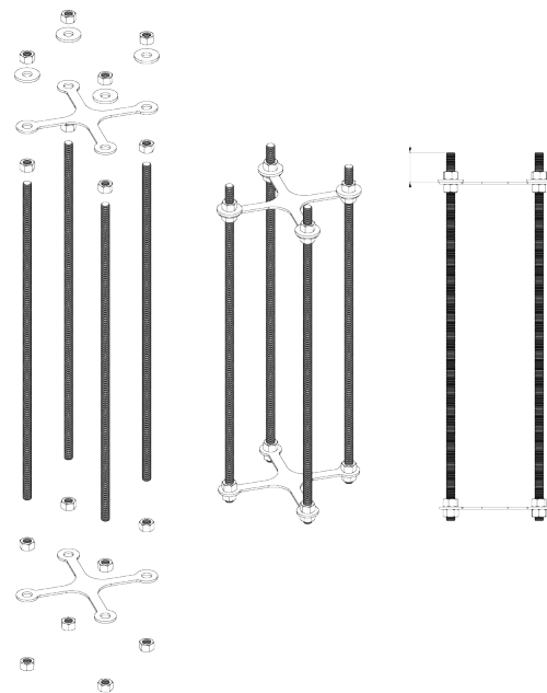
Rys. 25: Wytyczne do montażu zestawu fundamentowego Enelion.
