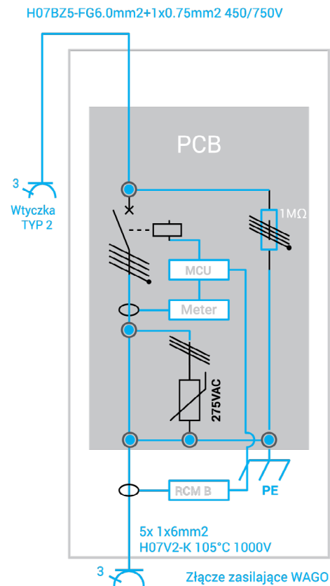
Rys. 17: Schematy poglądowe Modułów ENELION VERTICA część 2./2.
