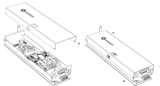
Rys. 64: Otwieranie modułu ENELION VERTICA.
