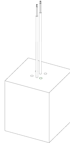
Rys. 22: Wykonane otwory pod kotwy chemiczne.
