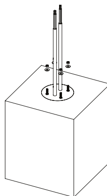
Rys. 32: Wkręcenie nakrętek i podkładek dystansowych na wystające pręty.
