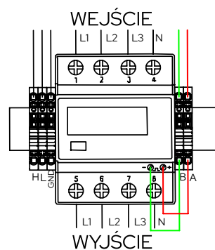
Rys. 45: Schemat podłączenia przewodów komunikacyjnych licznika MID dla słupa ENELION VERTICA wyposażonego w moduł ENELION VERTICA link.
