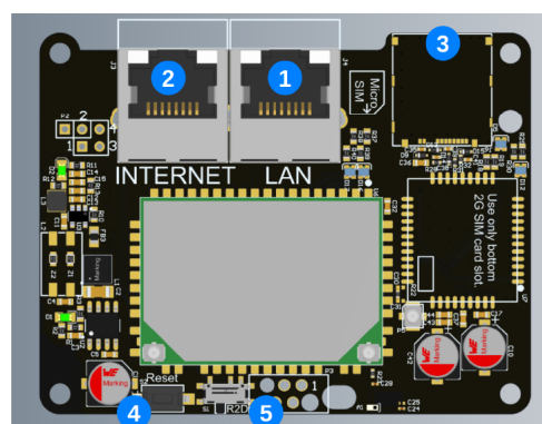
Rys. 48: Schemat modułu Enelion BRIDGE.
