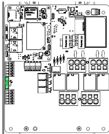
Rys. 71: Złącze komunikacyjne dodatku Enelion RCM B.
