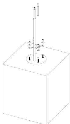
Rys. 31: Usunięcie górnej płyty bazowej z zestawu fundamentowego.
