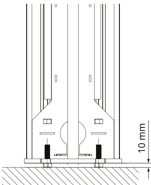
Rys. 35: Przekrój przez podstawę Słupa ENELION VERTICA podczas montażu.
