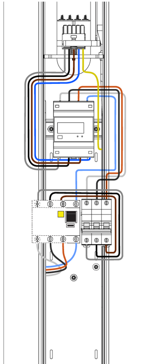
Rys. 62: Rewers Słupa ENELION VERTICA po zamontowaniu ENELION VERTICA Splitter z obecnym licznikiem MID.
