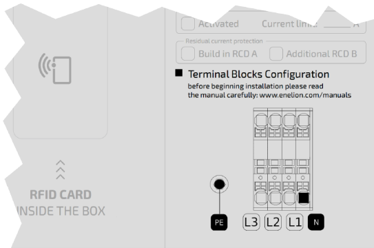
Rys. 37: Przykładowy fragment etykiety produktu.
