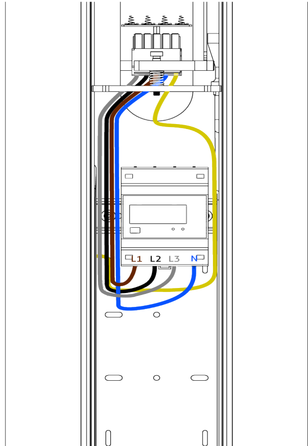
Rys. 40: Zamontowany licznik MID w Słupie ENELION VERTICA.
