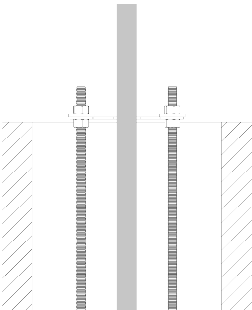
Rys. 27: Szczegóły umieszczenia górnej płyty bazowej w wykopie.
