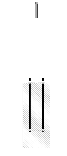
Rys. 29: Przekrój zabetonowanego zestawu fundamentowego.
