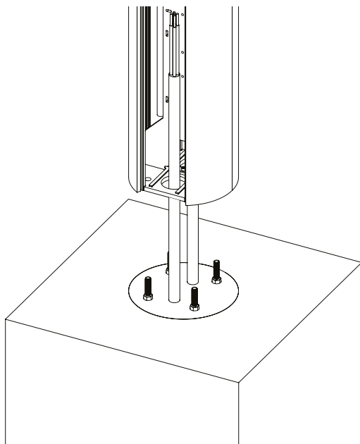
Rys. 34: Osadzanie Słupa ENELION VERTICA na fundamencie.
