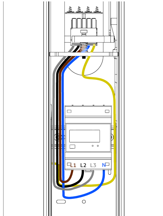
Rys. 43: Przykładowe podłączenie Słupa ENELION VERTICA z zastosowaniem licznika MID.
