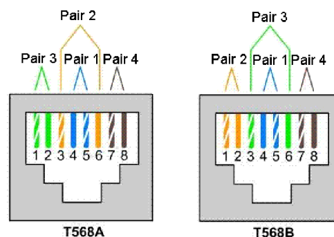
Rys. 46: Zakończenie przewodu Ethernet wg TIA-568A/B do 100BaseT.
