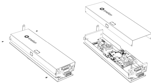
Rys. 73: Otwieranie Modułu ENELION VERTICA.
