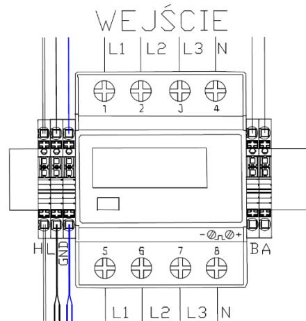
Rys. 53: Podłączenie przewodów komunikacyjnych (dla słupa ENELION VERTICA wyposażonego w moduł ENELION VERTICA link).
