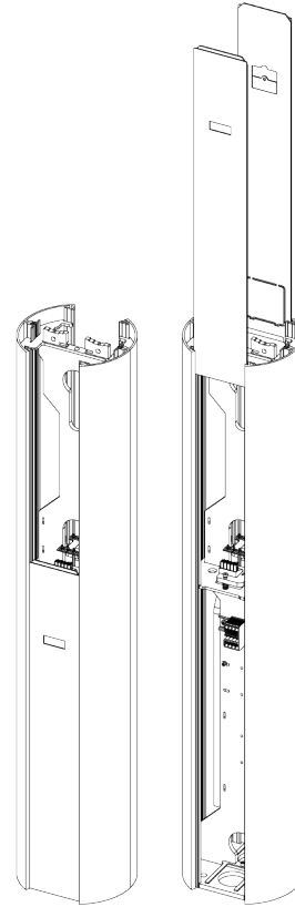
Rys. 33: Wysuwanie dolnych paneli maskujących ze Słupa ENELION VERTICA.
