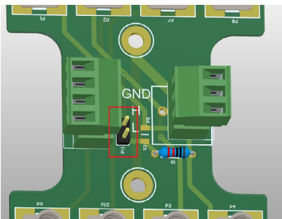
Rys. 57: Punkt zastosowania zworki terminującej.
