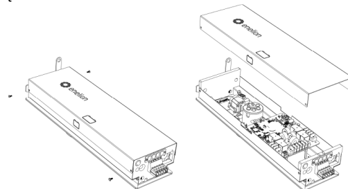
Rys. 68: Otwieranie Modułu ENELION VERTICA
