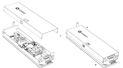
Rys. 72: Zamykanie Modułu ENELION VERTICA z RCM B.
