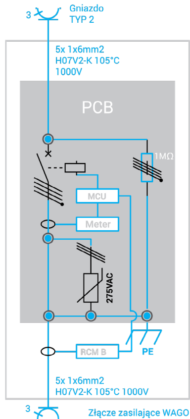
Rys. 17: Schematy poglądowe Modułów ENELION VERTICA część 2./2.
