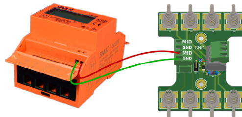
Rys. 44: Schemat podłączenia przewodów komunikacyjnych licznika MID dla słupa ENELION VERTICA wyposażonego w moduł ENELION VERTICAN.
