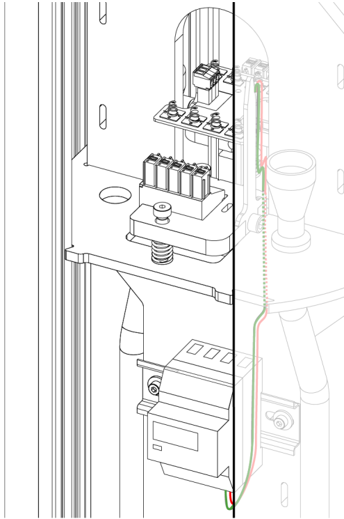
Rys. 41: Prowadzenie przewodów sygnałowych licznika MID w słupie wyposażonym w moduł VERTICAN
