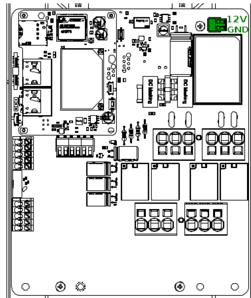
Rys. 75: Złącze dla przewodu zasilającego modułu LTE
