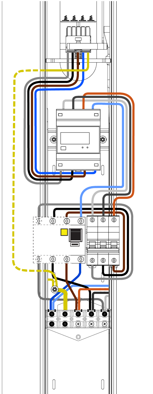
Rys. 61: Awers Słupa ENELION VERTICA po zamontowaniu ENELION VERTICA Splitter z obecnym licznikiem MID.
