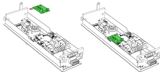
Rys. 65: montaż Enelion BRIDGE w module ENELION VERTICA.
