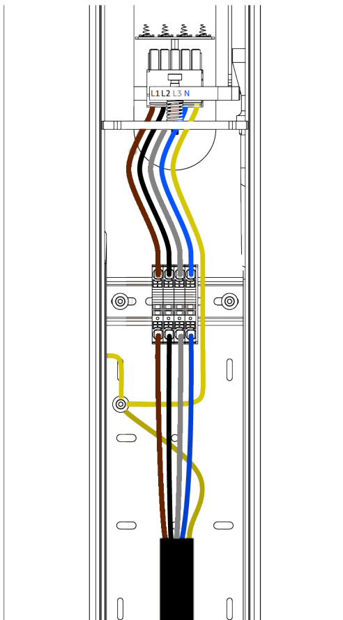
Rys. 38: Przykładowe podłączenie Słupa ENELION VERTICA.
