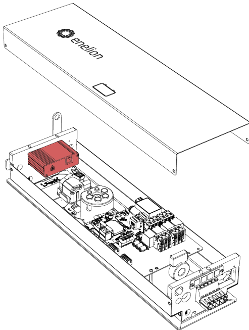
Rys. 74: Montaż modułu LTE.
