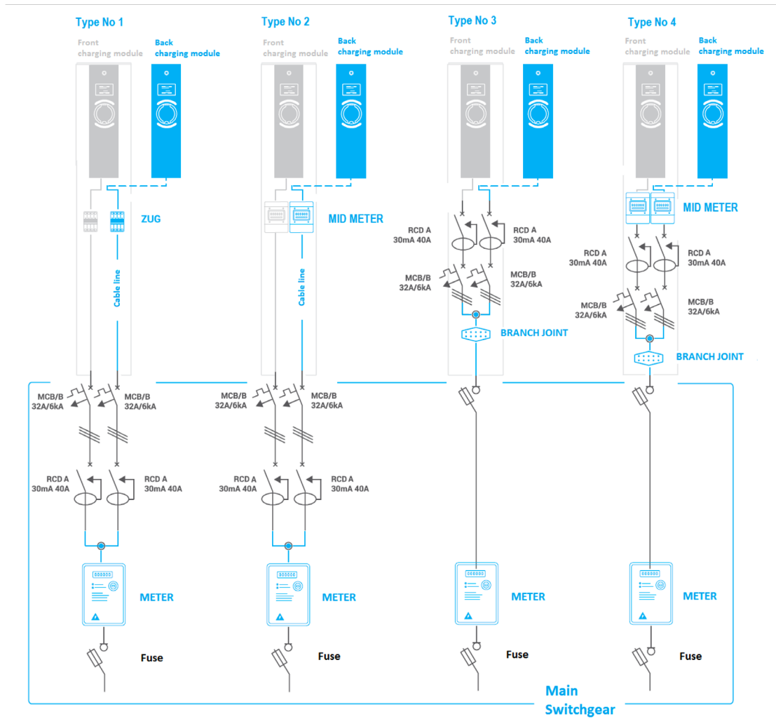
Rys. 14: Warianty podłączenia część 1./2.
