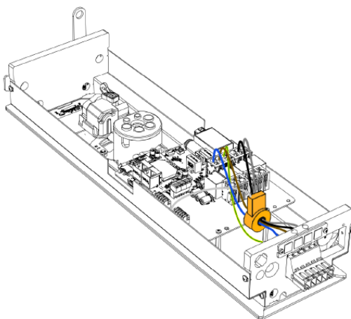
Rys. 70: Moduł ENELION VERTICA podczas montażu dodatku Enelion RCM B.
