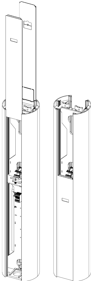
Rys. 63: Rewers Słupa ENELION VERTICA po zamontowaniu ENELION VERTICA Splitter z obecnym licznikiem MID.
