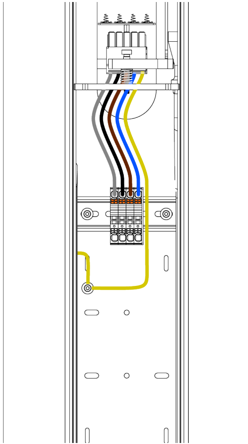
Rys. 39: Standardowe przyłącze Słupa ENELION VERTICA.
