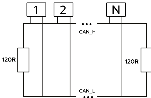
Rys. 55: Schemat terminacji magistrali komunikacyjnej.
