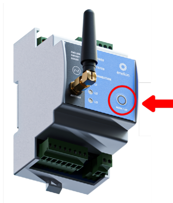
Rys. 16: Przycisk zmiany trybów połączenia
