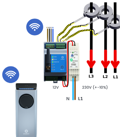
Rys. 5: Schemat podłączenia 3-fazowego wariantu ENELION ENERGY GUARDA
