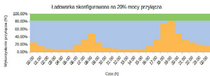
Rys. 14: Brak systemu DLB
