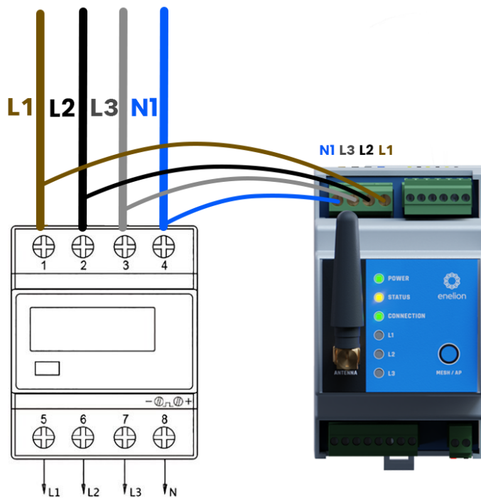
Rys. 6: Przykładowe podłączenie torów napięciowych do wybranego aparatu w rozdzielnicy
