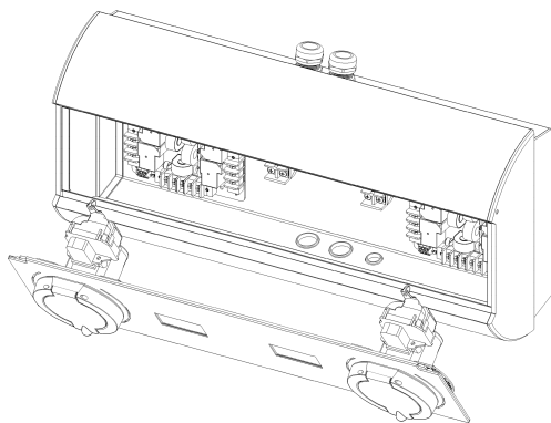
Rys. 9: Otwarte urządzenie z dostępem do wnętrza.
