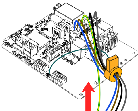
Rys. 27: Podłączenie RCM B.
