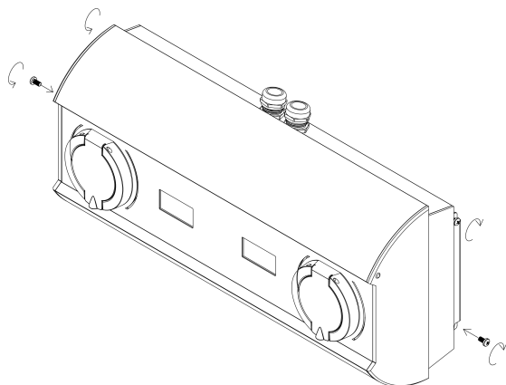
Rys. 14: Przykręcanie urządzenia do uchwytyów.
