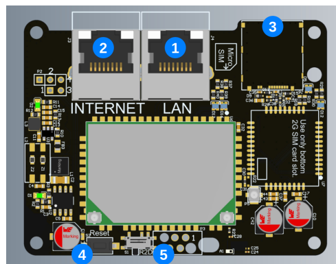
Rys. 37: Schemat modułu Enelion Bridge.
