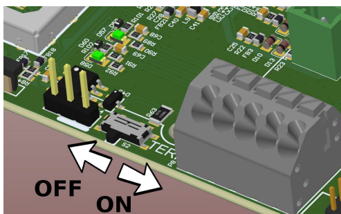
Rys. 35: Punkt zastosowania zworki terminującej (wariant B)
