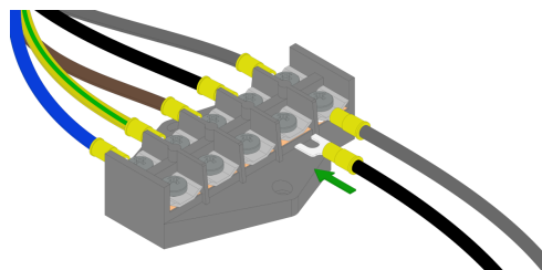
Rys. 21: Podłączenie z wykorzystaniem terminali widelkowych.
