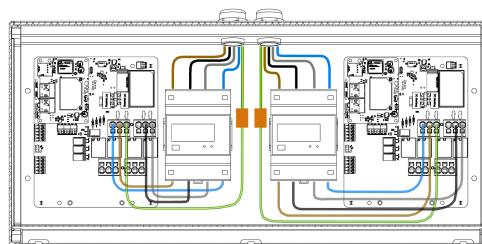
Rys. 24: Poprawnie wykonane podłączenie elektryczne z licznikami MID.
