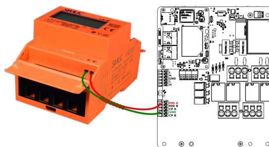
Rys. 25: Schemat podłączenia przewodów komunikacyjnych licznika MID.
