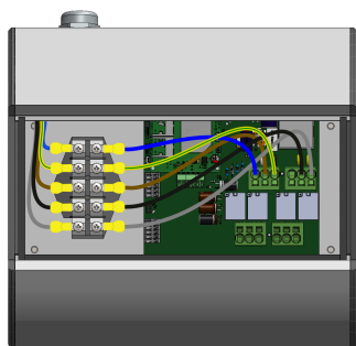
Rys. 20: Poprawnie wykonane podłączenie elektryczne.
