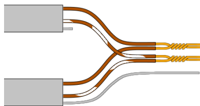
Rys. 25: Połączenie przewodu komunikacyjnego wchodzącego z wychodzącym (wariant A)
