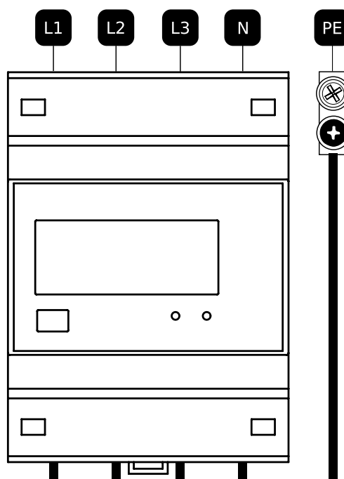
Rys. 21: Wytyczne podłączenia przy stosowaniu licznika MID.
