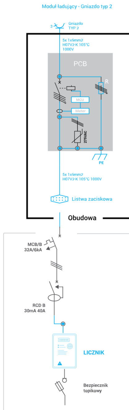
Rys. 16: Schematy wariantów podłączenia 1./2.
