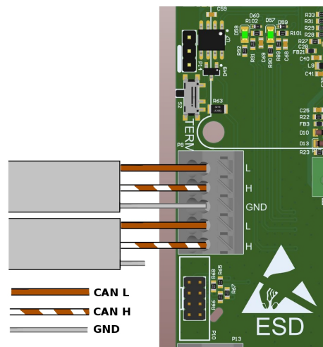
Rys. 28: Schemat podłączenia przewodów komunikacyjnych Enelion Chain (wariant B)
