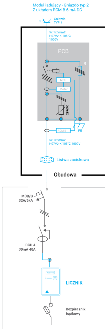
Rys. 16: Schematy wariantów podłączenia 1./2.
