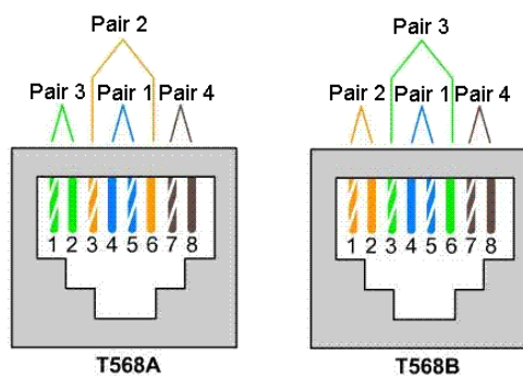
Rys. 33: Zakończenie przewodu Ethernet wg TIA-568A/B do 100BaseT.
