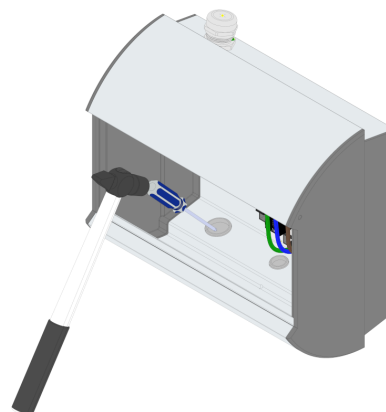
Rys. 12: Usuwanie zaślepień wpustów kablowych.
