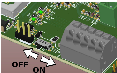
Rys. 32: Punkt zastosowania zworki terminującej (wariant B)
