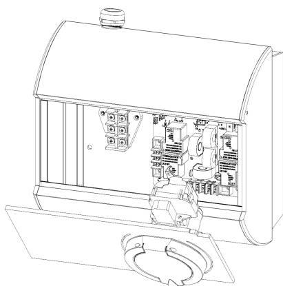
Rys. 8: Otwarte urządzenie z dostępem do wnętrza.
