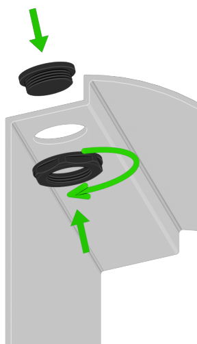
Rys. 15: Sposób montażu dodatkowej zaślepki.
