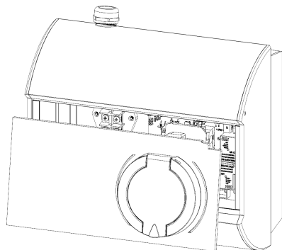
Rys. 7: Wyciąganie panelu przedniego.
