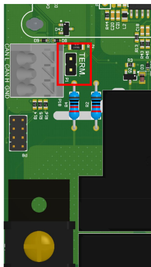
Rys. 31: Punkt zastosowania zworki terminującej (wariant A)
