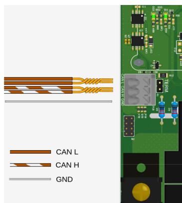
Rys. 27: Schemat podłączenia przewodów komunikacyjnych Enelion Chain (wariant A)
