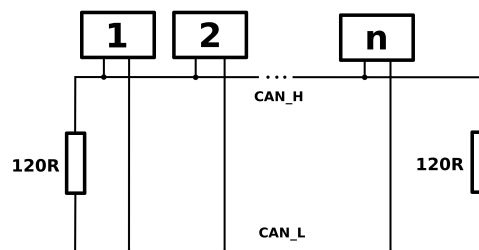
Rys. 29: Schemat terminacji magistrali komunikacyjnej.
