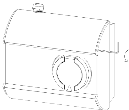
Rys. 3: Wykręcanie trzpienia blokującego.
