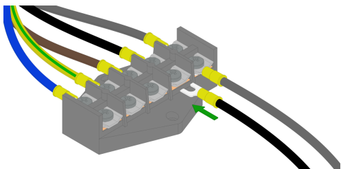
Rys. 18: Podłączenie z wykorzystaniem terminali widelkowych.
