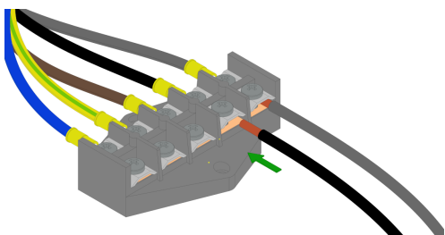
Rys. 19: Podłączenie z wykorzystaniem żył pełnych - drut.
