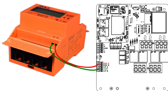
Rys. 22: Schemat podłączenia przewodów komunikacyjnych licznika MID.
