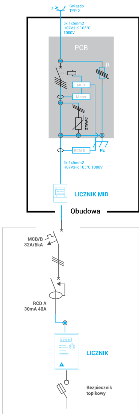
Rys. 17: Schematy wariantów podłączenia 2./2.
