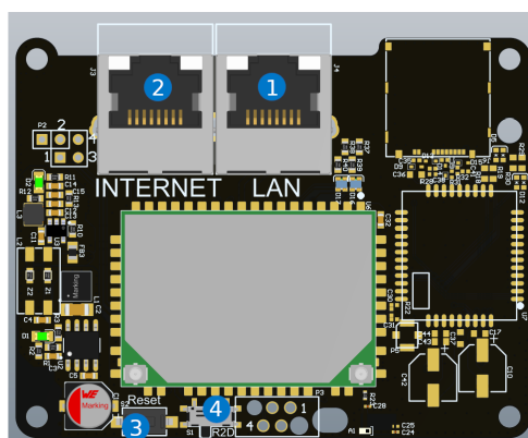
Rys. 34: Schemat modułu Enelion Bridge.
