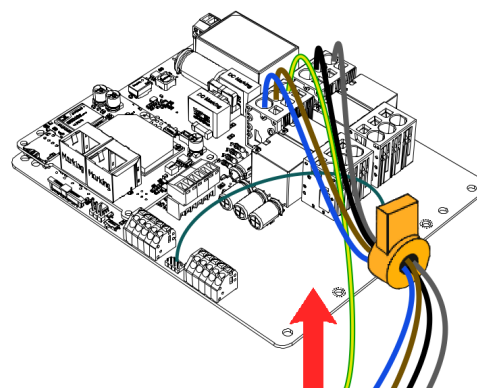
Rys. 24: Podłączenie RCM B.
