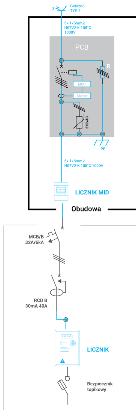
Rys. 17: Schematy wariantów podłączenia 2./2.
