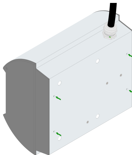
Rys. 10: Otwory montażowe Enelion Wallbox widoczne od tyłu urządzenia.
