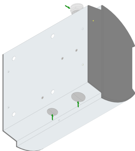
Rys. 11: Pozycje punktów wprowadzania przewodów w Enelion Wallbox.
