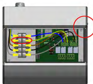
Rys. 48: Główny Punkt Wyrównawczy stacji Wallbox
